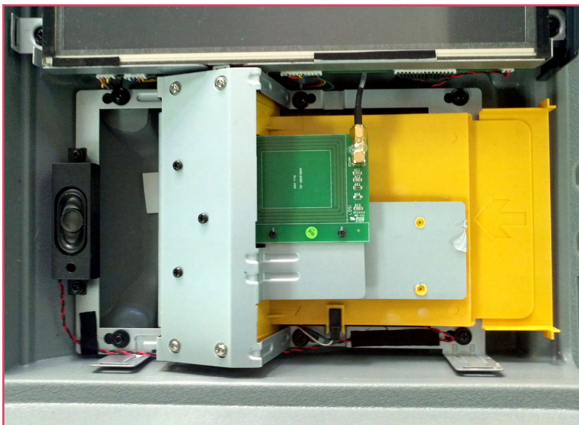
FIGURA 7: Impresora térmica y lector/grabador RFID
