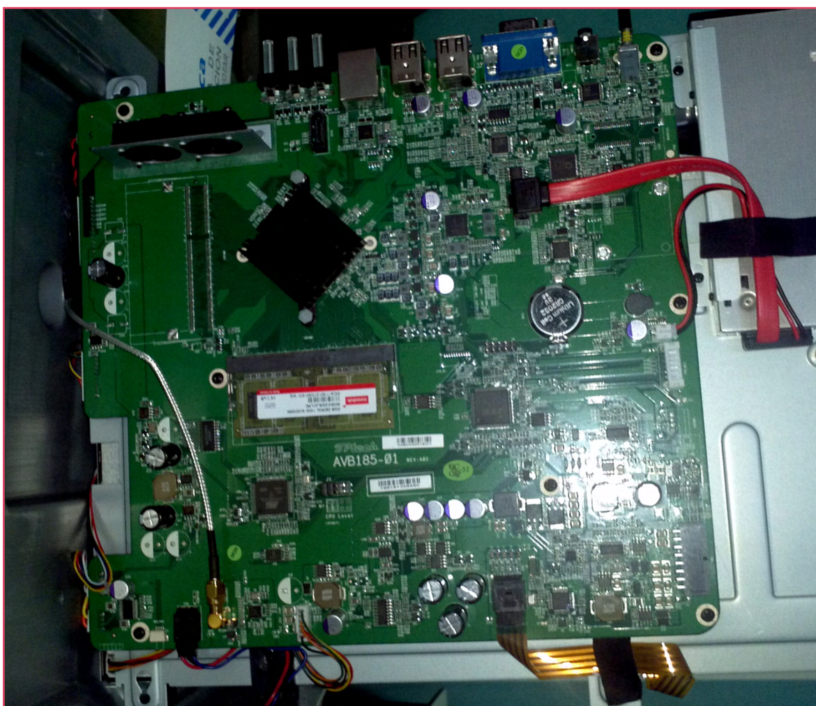
FIGURA 5: Placa base
